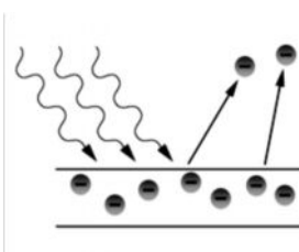
Рисунок 1. Иллюстрация испускания фотоэлектронов с поверхности металлической пластины.
