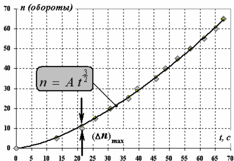
График 9. Закон движения (степенная зависимость)
