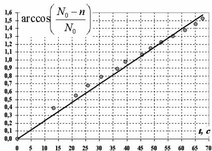
График 6. Модель гармонического колебания (Линеаризация)
