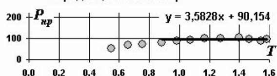
Нерадиационные потери
