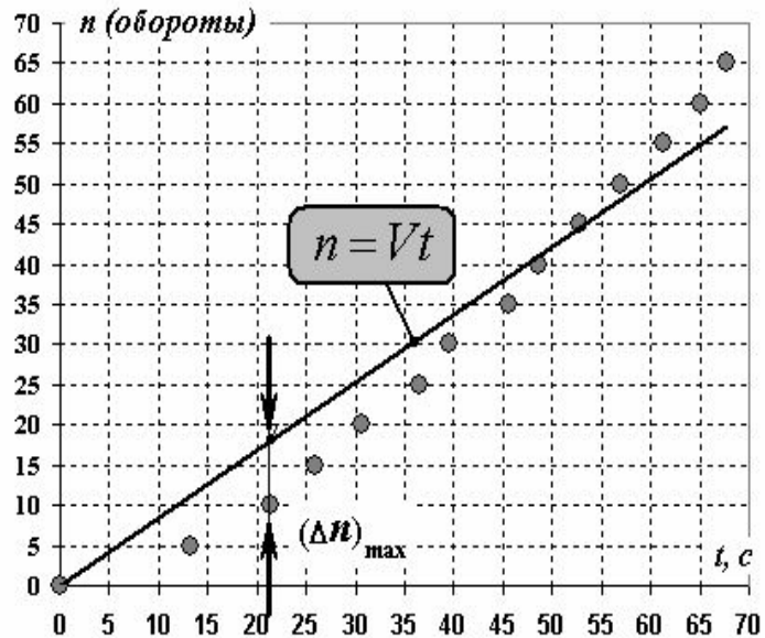
График 2. Закон движения (модель равномерного движения)
